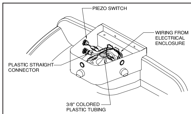
Piezo Push Button
